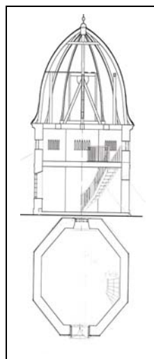
23. Griezums un plāns
