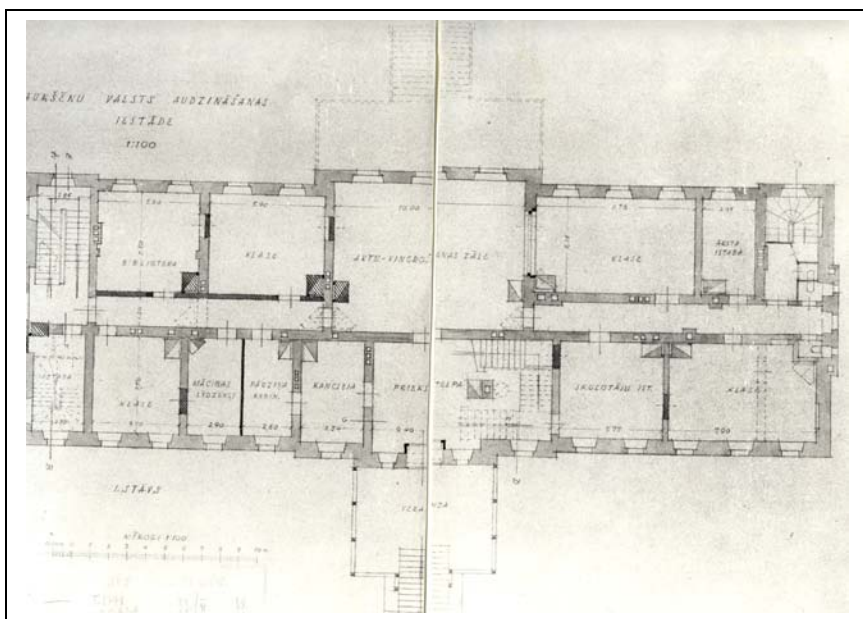
18. Pils pārbūves projekts. 1938.g. (LVVA)
